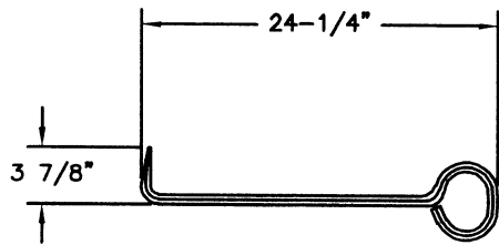
PULHEXFLAT
