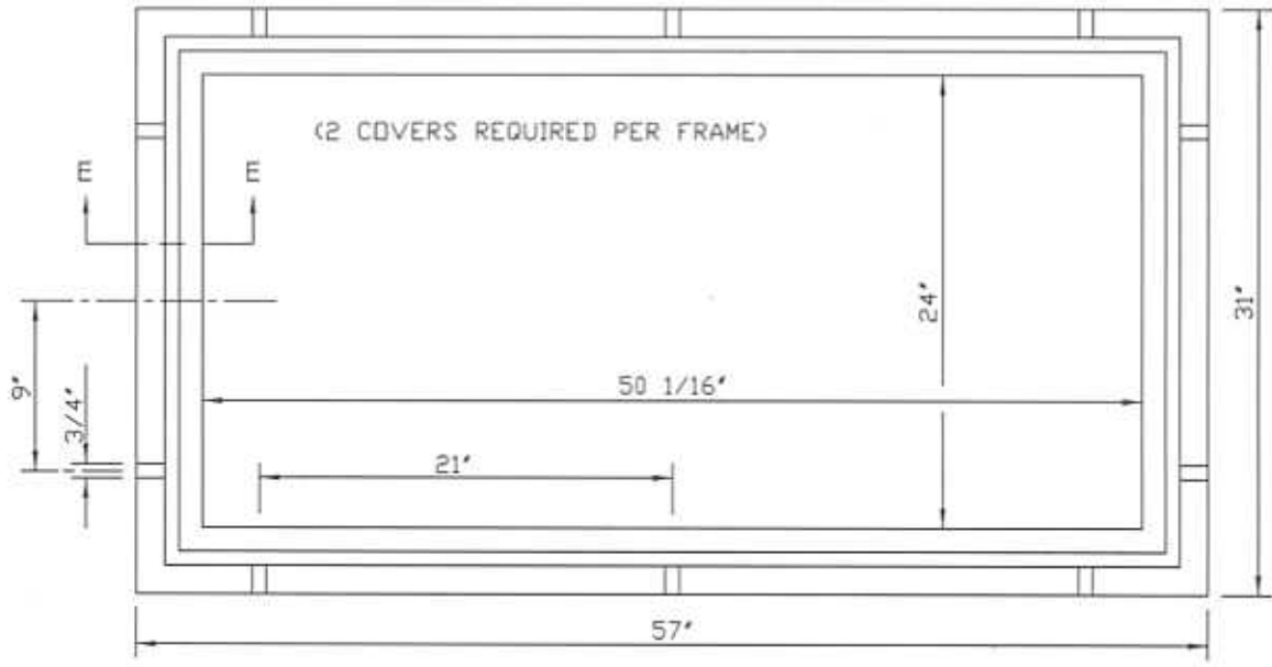
MANHOLE FRAME
