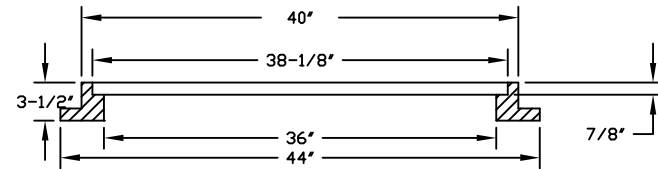
MANHOLE RING
